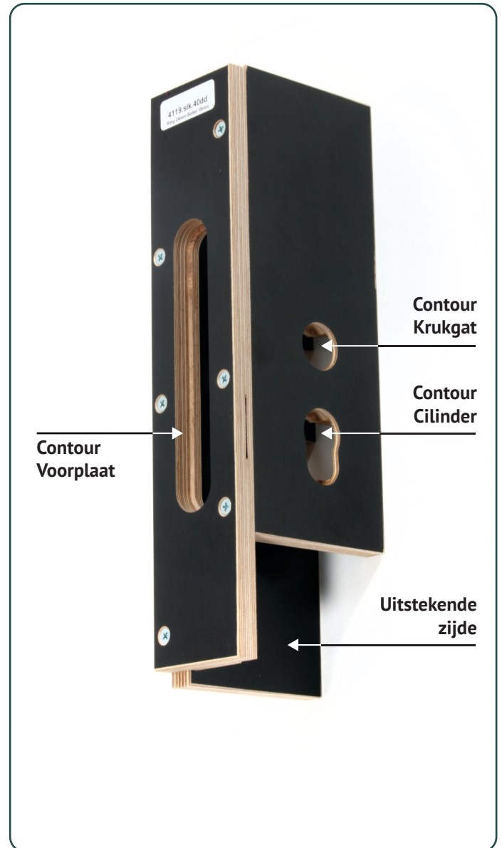
Afb. 1 - Slotkast freesmal
