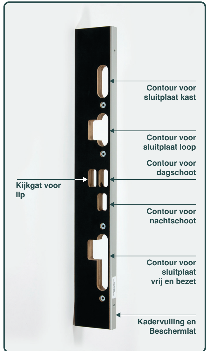
afb. 1 - Sluitplaat freesmal
